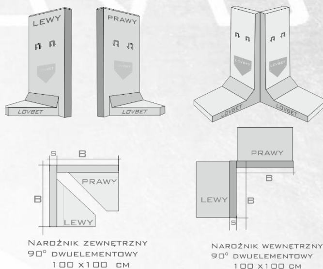
Rys. 7. Narożniki murów oporowych
